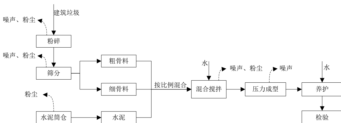
图 2-3 工艺流程及产污环节图
