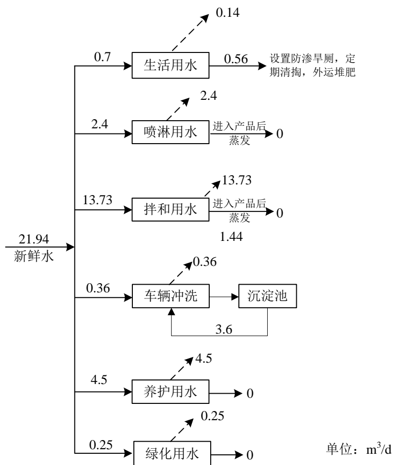
图 2-2 水平衡图 单位: m 3 /d
